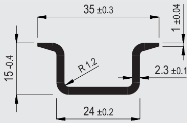
nach EN 60715
